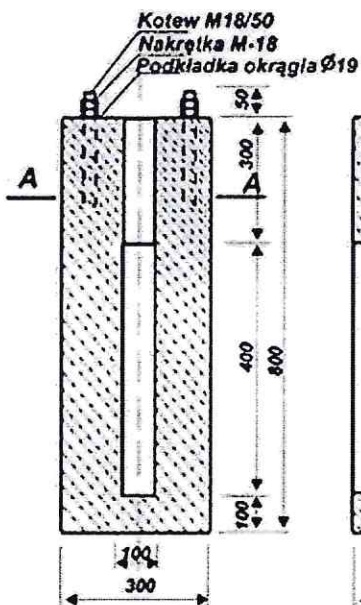
Przekrój B-B
